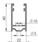
Nákres vrtání děr vodící lišty.
