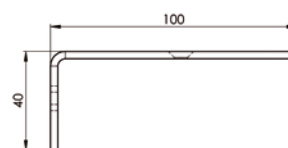
Konzola L (RO-018, 7-302233)
